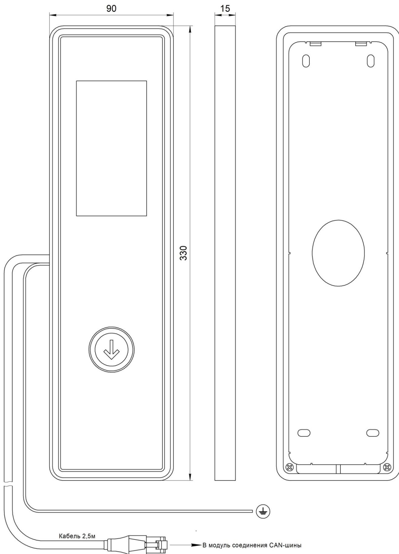
Рис.1 Внешний вид, габаритные и установочные размеры Вызывного поста ОБСИДИАН (жгут RJ45) НШЕК.468381.227-01
